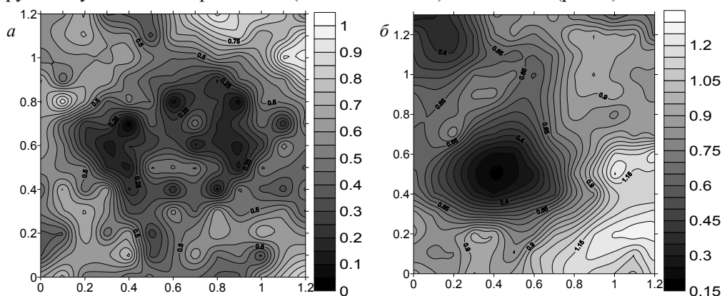
Рис. 1. Электрическая проводимость почвы в пределах одного пороя (дС/м): а – порой 1, б – порой 2
