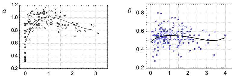
Рис. 5. Изменение электропроводности (дС/м) по мере удаления от центра поры (ось абсцисс, м) в пределах полигона: a – полигон 1, b – полигон 2
