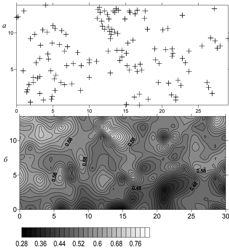
Рис. 4. Расположение поров на полигоне 2 ( a ) и электрическая проводимость почвы ( b , дС/м)
