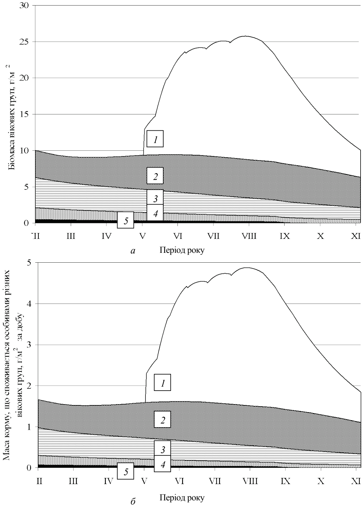
Рис. 3.3. Модель популяції R. kessleri :
