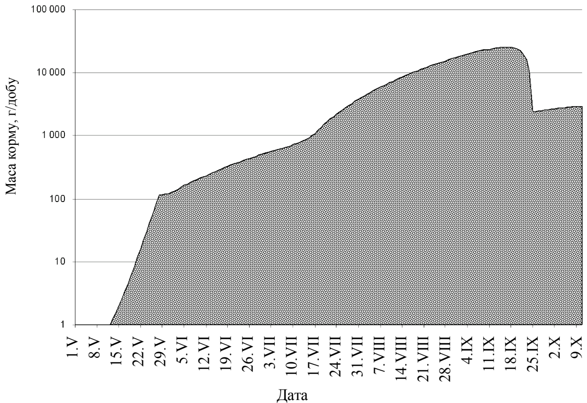
Рис. 2.5. Динаміка добового споживання корму популяцією L. decemlineata з рівномірним притоком особин (1 екземпляр за добу починаючи з 10 травня)
