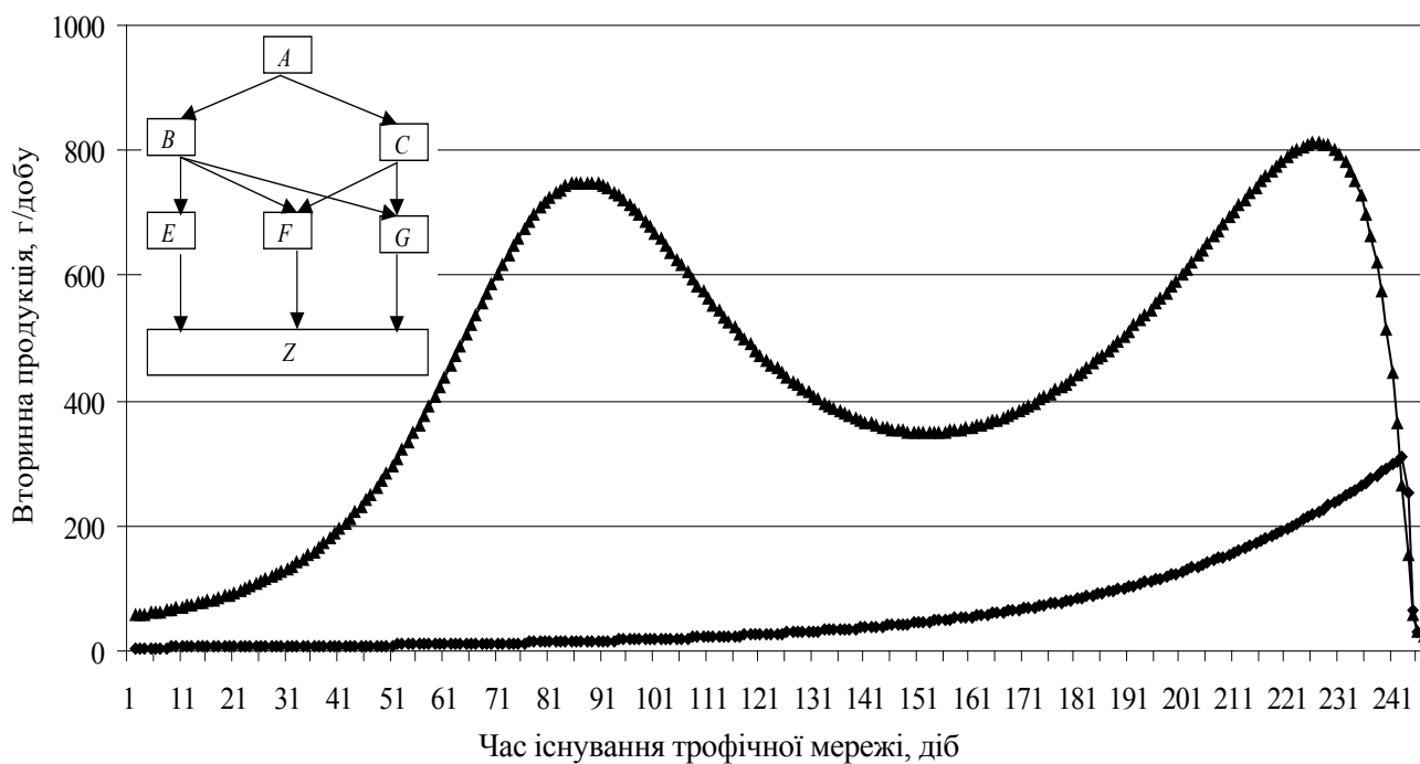
Рис. 4.7. Динаміка створення вторинної продукції у трофічній мережі (6 видів) за оптимальних початкових параметрів:
