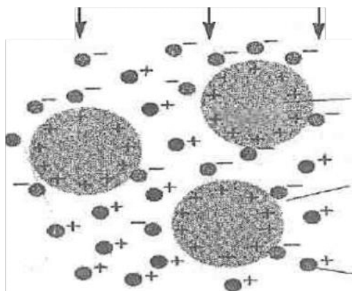
Рис. 5. Схематичне зображення розділення речовин методом іонообмінної хроматографії
